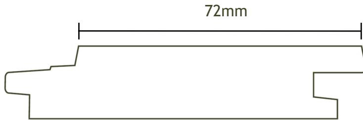
80 x 19 IRONOAK
